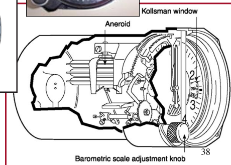
Altimeter
